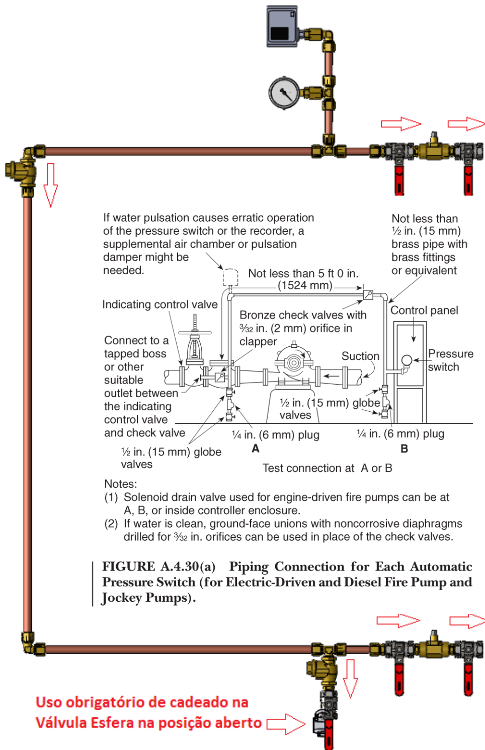
Cavalete de automação ( Linha sensível de pressão ) conforme NFPA-20 ed. 2013 ( Figura A.4.30(a) )
