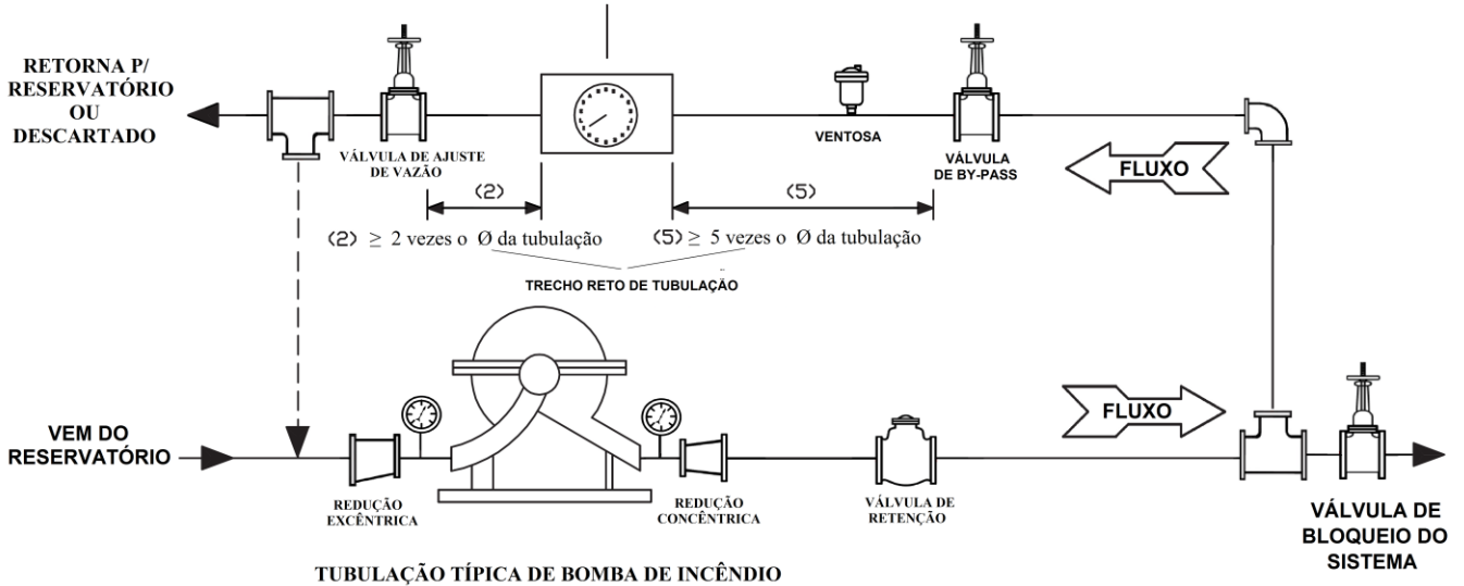
TUBULAÇÃO TÍPICA DE BOMBA DE INCÊNDIO
